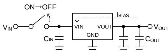
Figure 266. Open VIN
