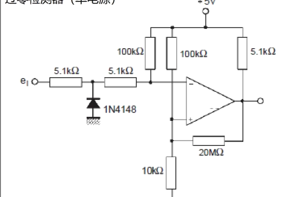
过零检测器 (单电源)
